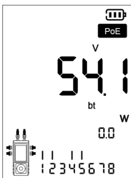
bt 协议 pin1/2 (+) 3/6 (-) 4/5 (+) 7/8 (-)
