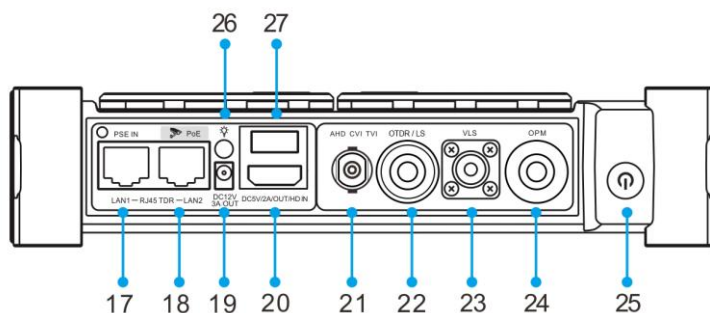
底部介面圖
