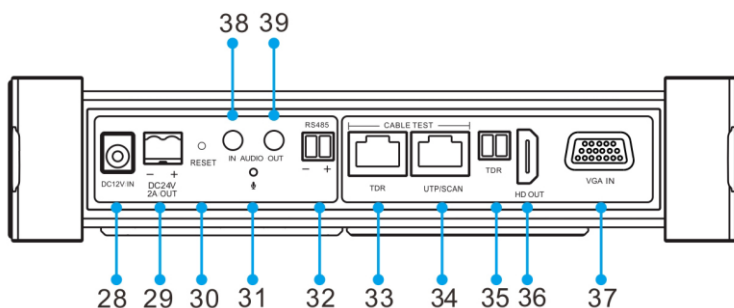
側面介面圖
